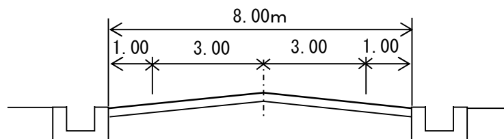
標準図（A）
