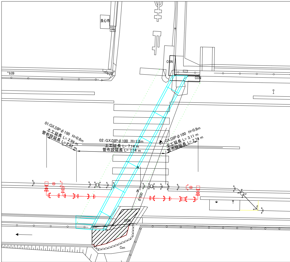
平面図
