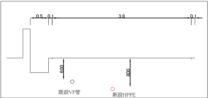
B-B'断面図
