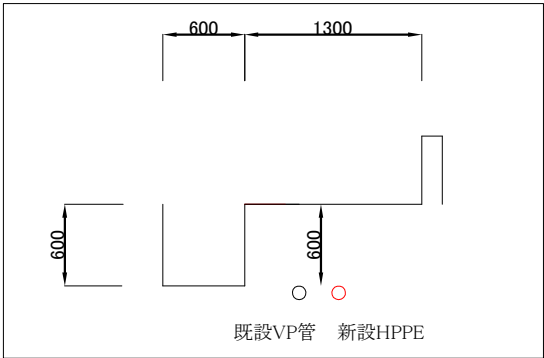
B-B'断面図
