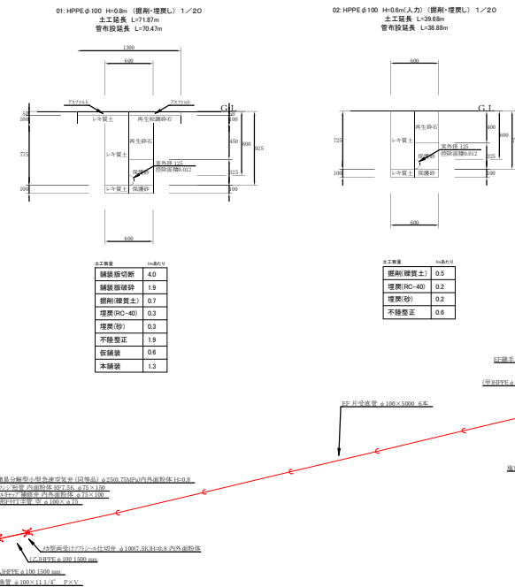
土工断面図
