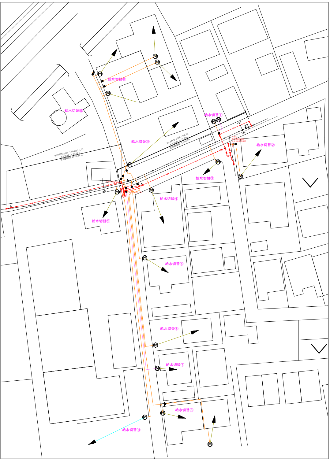
給水平面図
